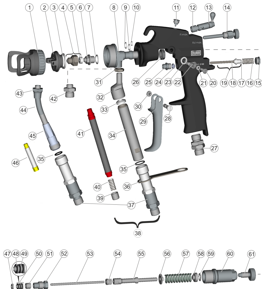
Fig. 27: EcoGun 2100
